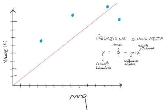
Figura 1.14 Nella figura è rappresentato l'algoritmo di regressione lineare con un esempio che ha come caratteristica i metri quadri di una casa e come variabile indipendente il suo valore.
