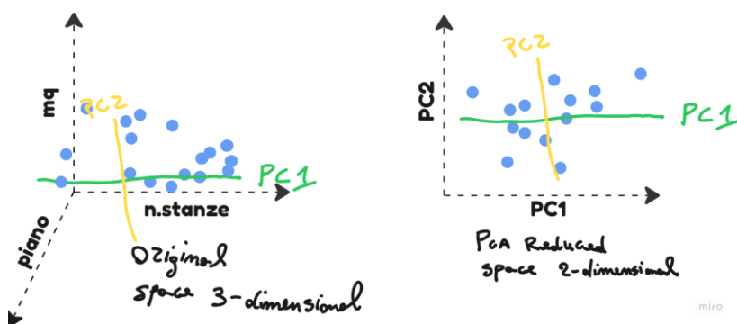
Figura 1.7 Riduzione delle feature grazie al PCA, lo schema a sinistra presenta 3 dimensioni numero di stanze, piano e mq, mentre quella a destra 2 dimensioni, ovvero PC1 e PC2 che PCA ha calcolato.
